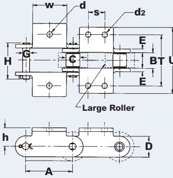
K-1 (Bent Lug 2 Sides - 1 Hole) K-2 (Bent Lug 2 Sides - 2 Holes)
