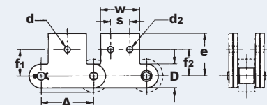
SK-1 (Straight Lug 2 Sides - 1 Hole) SK-2 (Straight Lug 2 Sides - 2 Holes)
