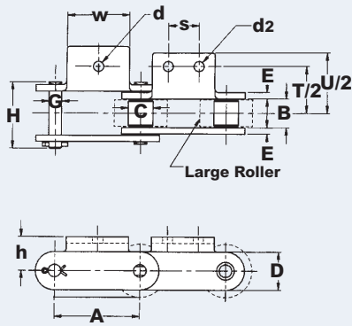
A-1 (Bent Lug 1 Side - 1 Hole) A-2 (Bent Lug 1 Side - 2 Holes)
