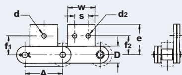
SA-1 (Straight Lug 1 Side - 1 Hole) SA-2 (Straight Lug 1 Side - 2 Holes)
